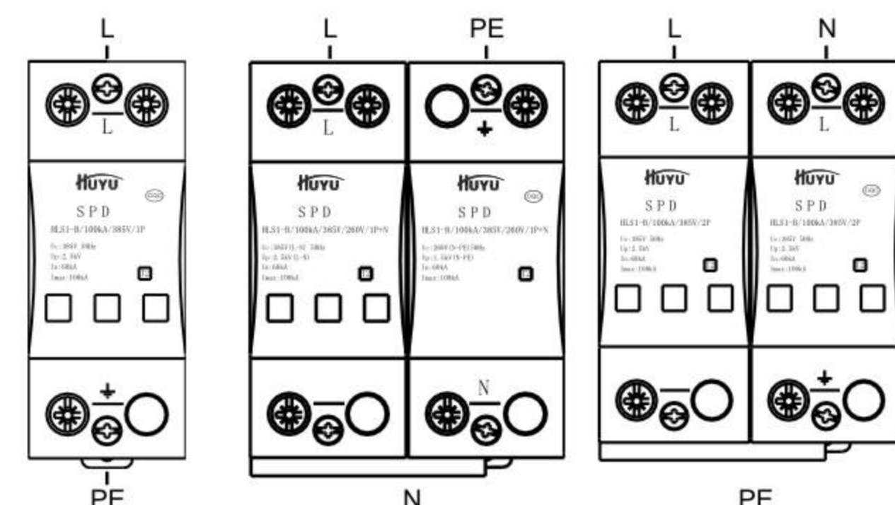
图2 电涌保护器的接线型式
