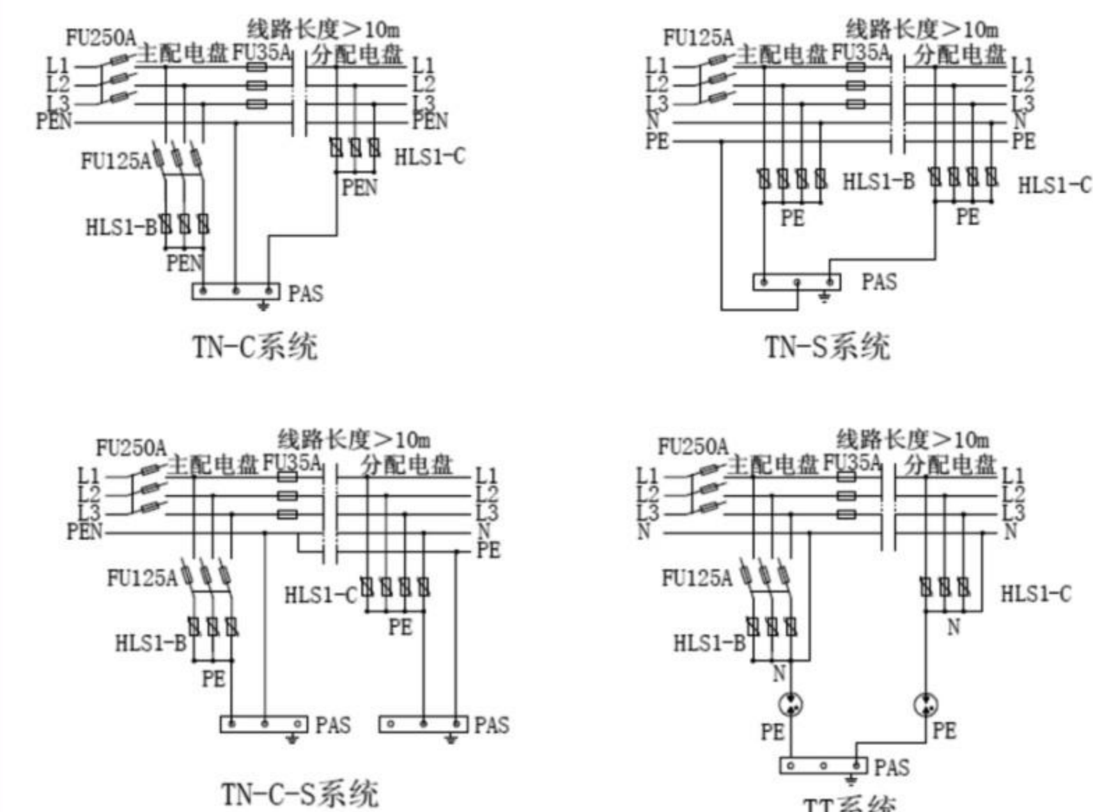
图1 TN-C、TN-S、TN-C-S及TT系统接线原理图
