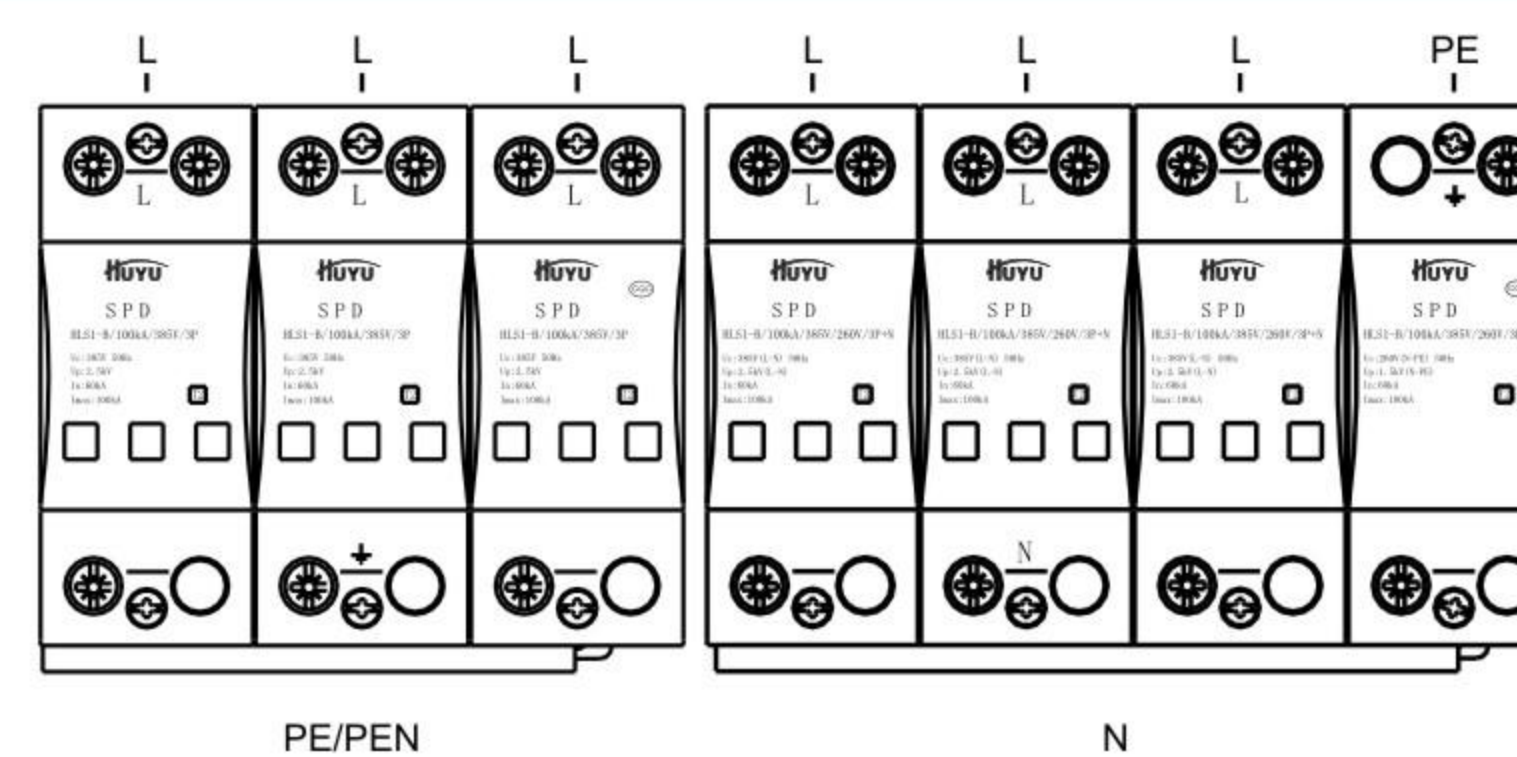
图2 (续) 电涌保护器的接线型式
